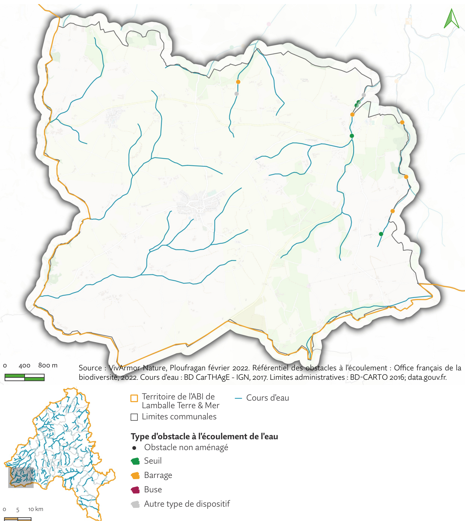
Carte B4c-1 : Obstacles à l'écoulement référencés sur la commune de Plémy
