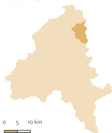
Carte B7-1 : Loutre d'Europe et évaluation du risque de collision routière des ouvrages hydrauliques sur la commune de Hénanbihen
